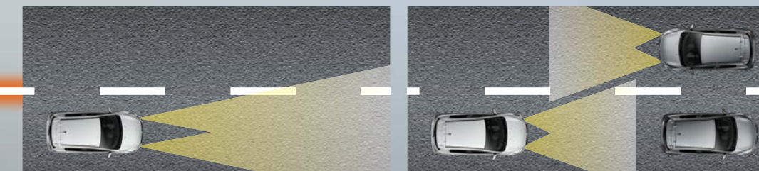
מערכת לשליטה אוטומטית על אורות גבוהים* Automatic High Beam - AHB
